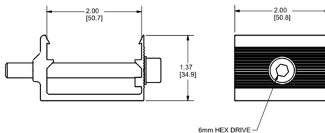
SMR 200 L-Foot Adaptor
