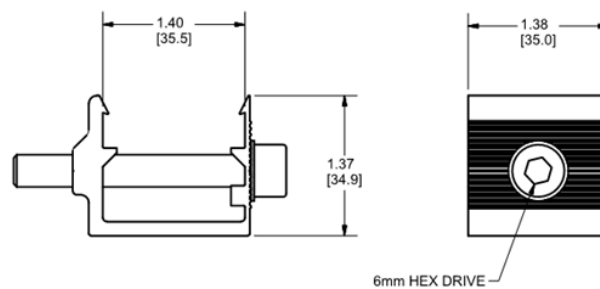
SMR 100 L-Foot Adaptor
