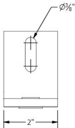
L-FOOT
